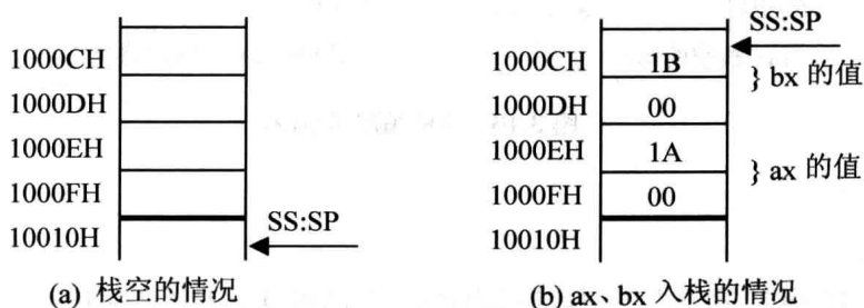
图 3.15 栈的情况示意(1)
