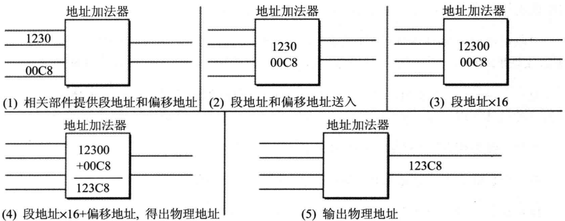
图 2.7 地址加法器的工作过程
