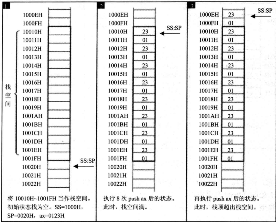
图 3.13 执行 push 后栈顶超出栈空间
