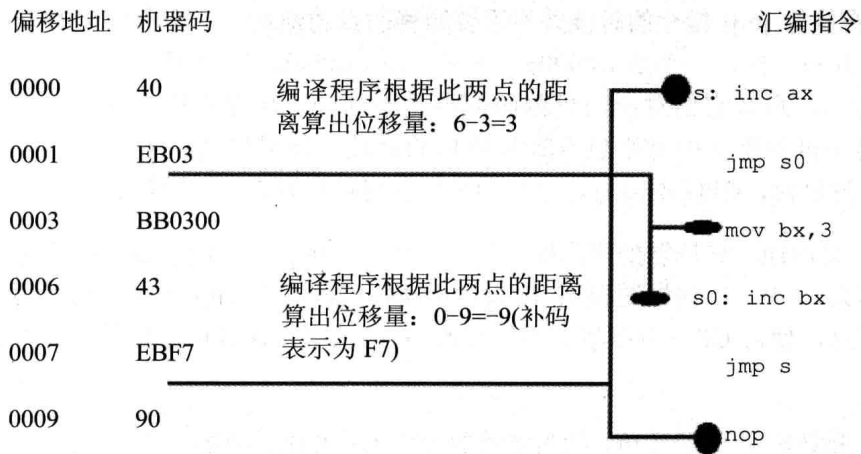
图 9.3 转移位移的计算方法
