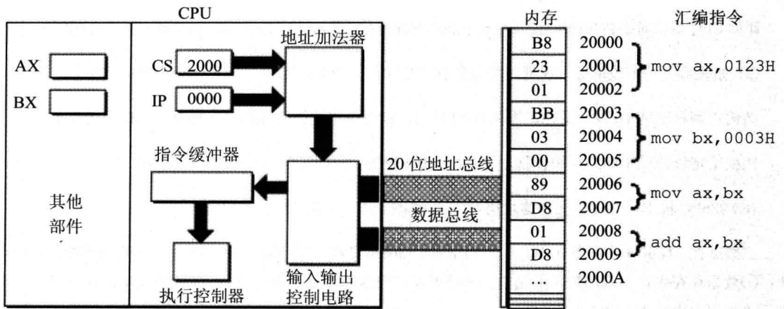
图 2.10 8086PC 读取和执行指令的相关部件
