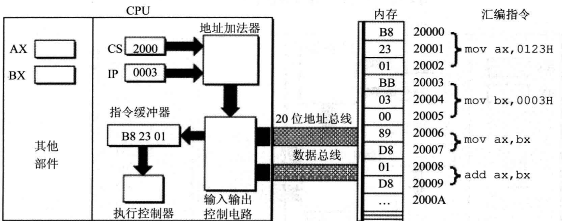
图 2.17 IP 中的值自动增加
