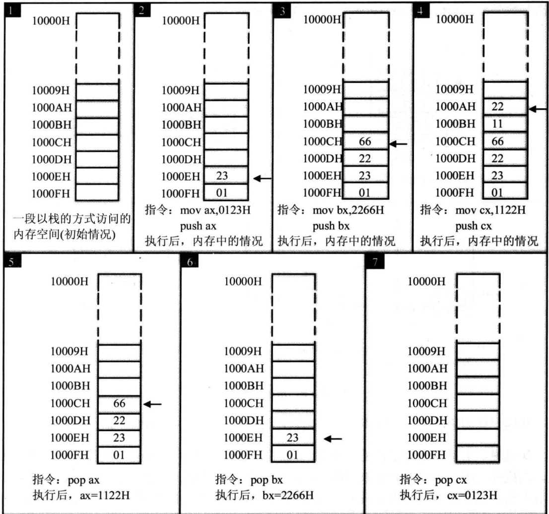
图 3.9 8086CPU 的栈操作
