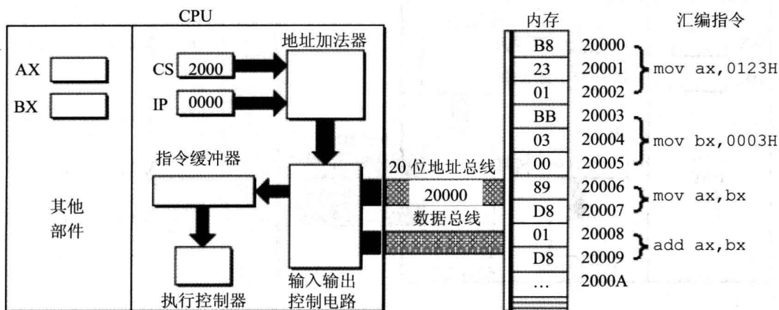
图 2.14 输入输出控制电路将物理地址 2000H 送上地址总线
