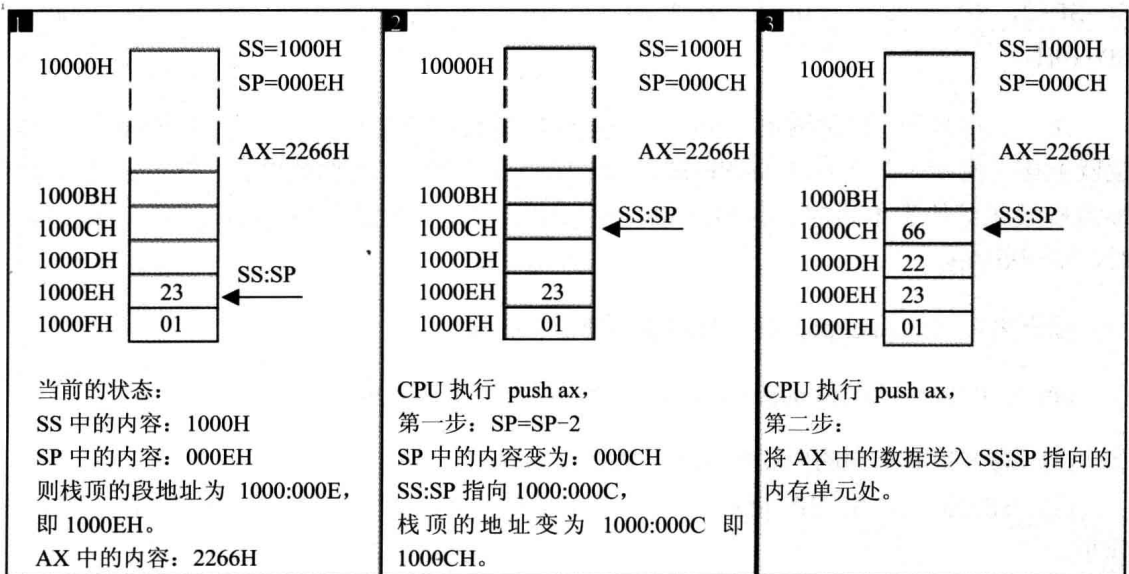
图 3.10 push 指令的执行过程
