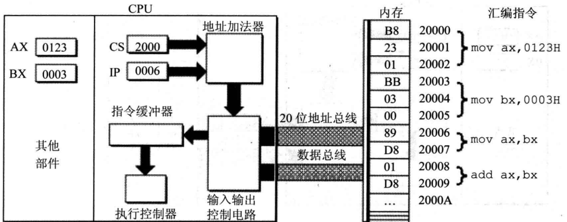
图 2.22 执行指令 BB 03 00(即 mov bx,0003H)
